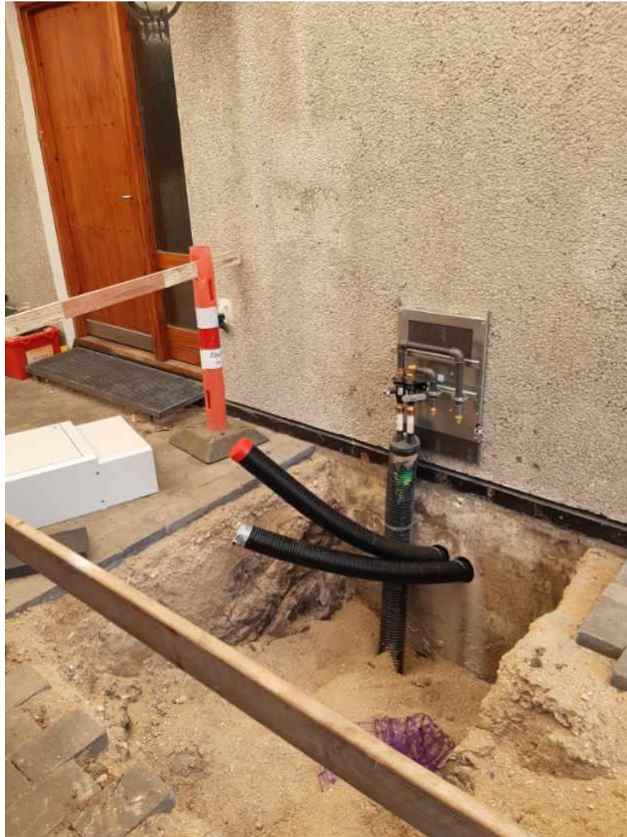
Løsning fra Poppelhusene i Avedøre
